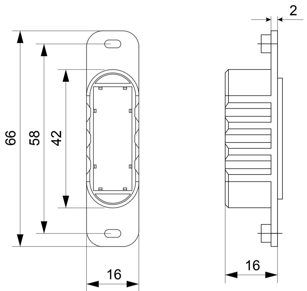
Пластиковая вставка под ответную планку
